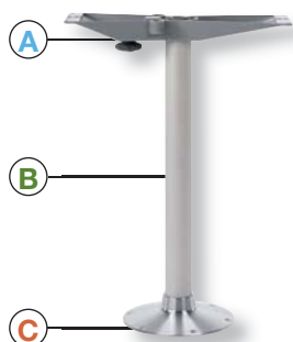
Vast tafelonderstel Ø 60 mm 1-zijde conisch Fixed table pedestal Ø 60 mm 1-side tapered
