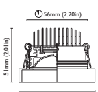
JACK 1 - 70 8W
