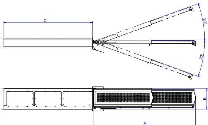
DIMENSIONI DELLA CASSA
