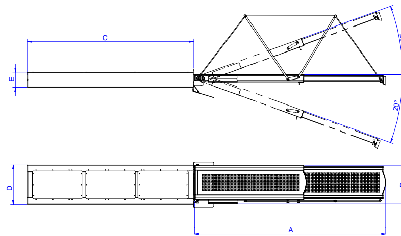
DIMENSIONI DELLA CASSA
